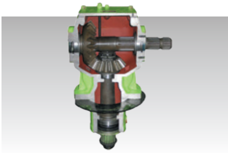
210PS starke Mulchgetriebe
