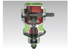
225PS Mulchgetriebe
