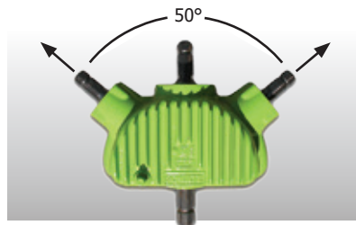
50° Verteilergetriebe für kurze Antriebsstränge
